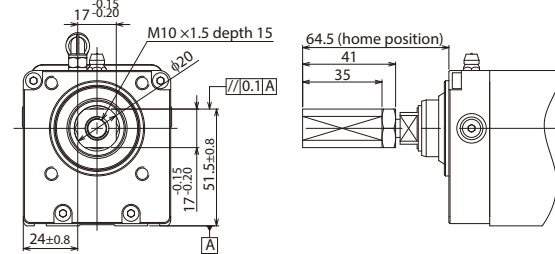
RCP6(S)W-RAA6□ Model Name: RCP6W-NFA-RAA6
